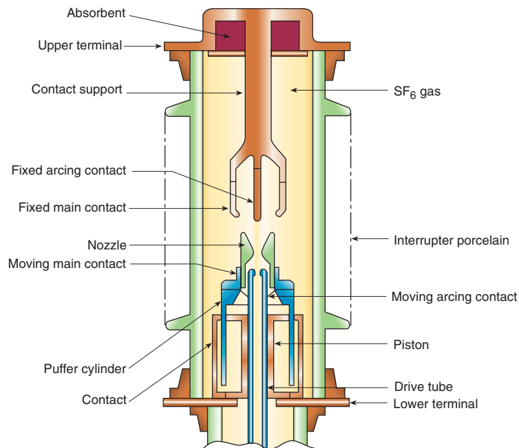
FIG. 2 : Open position
